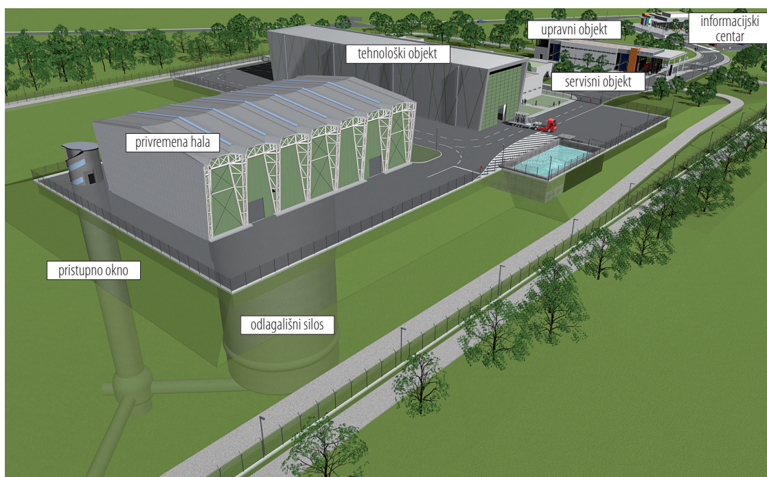
Ilustracija 1 Buduće odlagalište sa silosom za odlaganje u dubini zemlje
